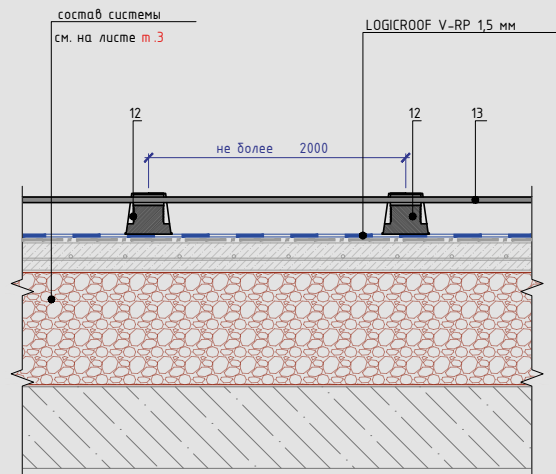
Устройство молниезащиты
